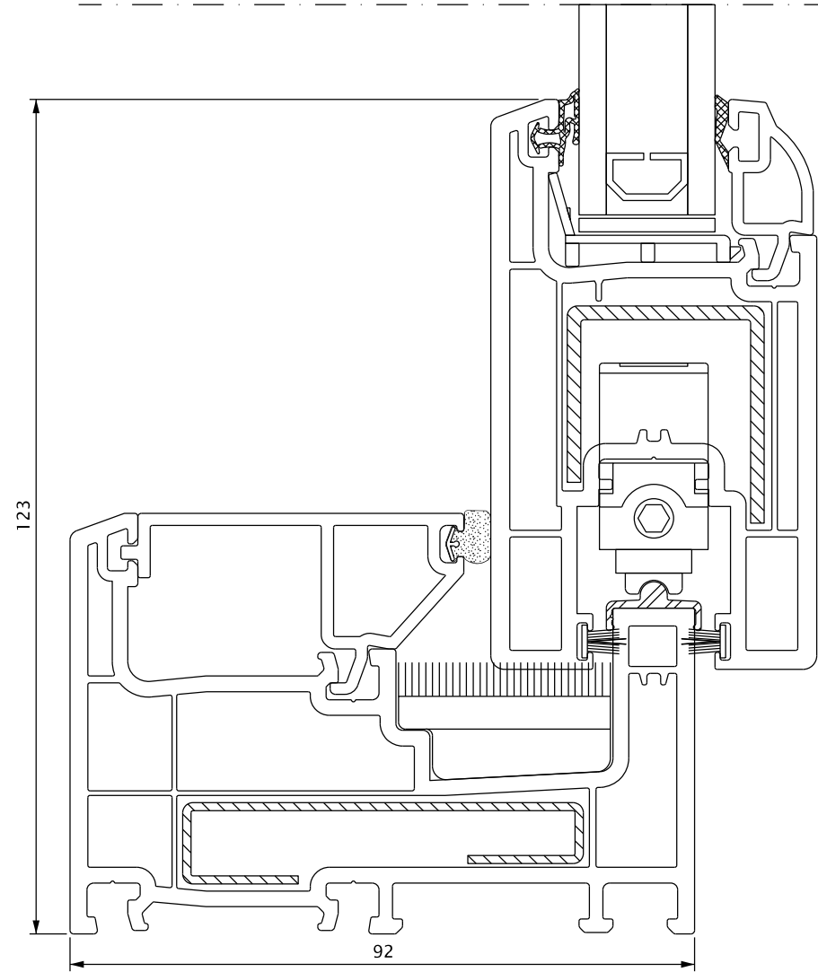
SBT.BLM. SÜRME KASA SÜRME KANAT FIXED SLIDING FRAME SLIDING SASH
